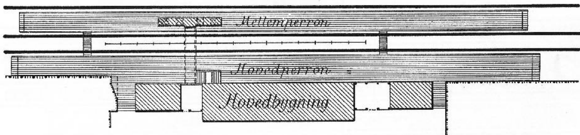
Fig. 110. Station med hovedspor og dobbeltsidet mellemperron.
